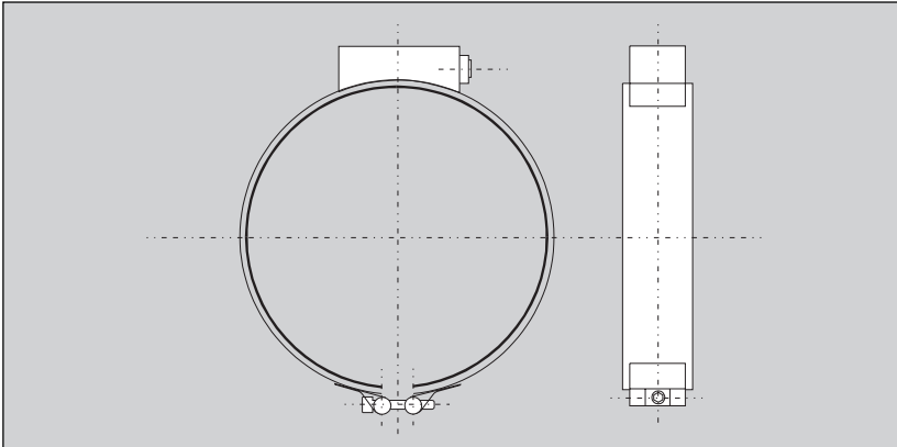
Das Glimmerheizband (Typ GHB) für Betriebstemperaturen bis maximal 350 °C
